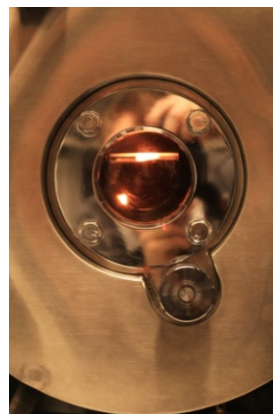
Bild 4 visar sintringskammaren
